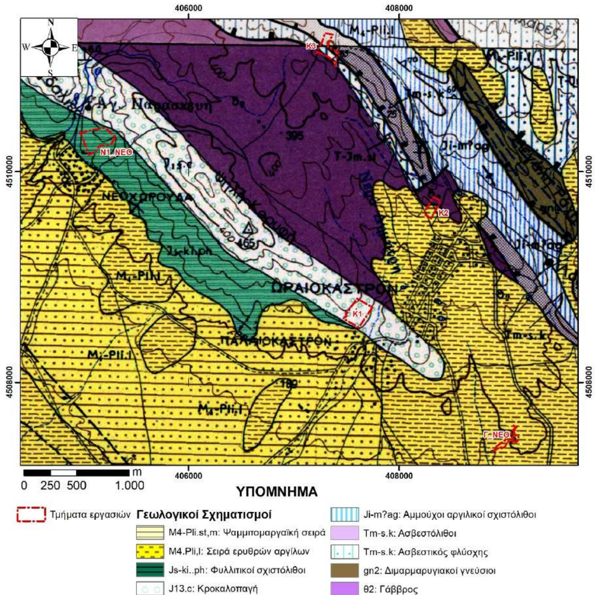
Εικόνα 4: Γεωλογικός χάρτης της υπό μελέτη περιοχής (Πηγή: Γεωλογικός χάρτης ΙΓΜΕ, Φύλλα Χάρτη Θεσσαλονίκης και Κιλκίς).
