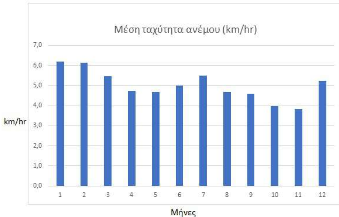
Γράφημα 3: Μακροχρόνια δεδομένα ταχύτητας ανέμου για το Κορδελιό (Πηγή: meteo.gr).
