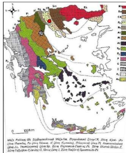
Εικόνα 3: Σχηματική απεικόνιση της Γεωτεκτονικής του Ελλαδικού χώρου (Ελληνίδων Ζωνών). Εντοπίζεται η περιοχή μελέτης.
