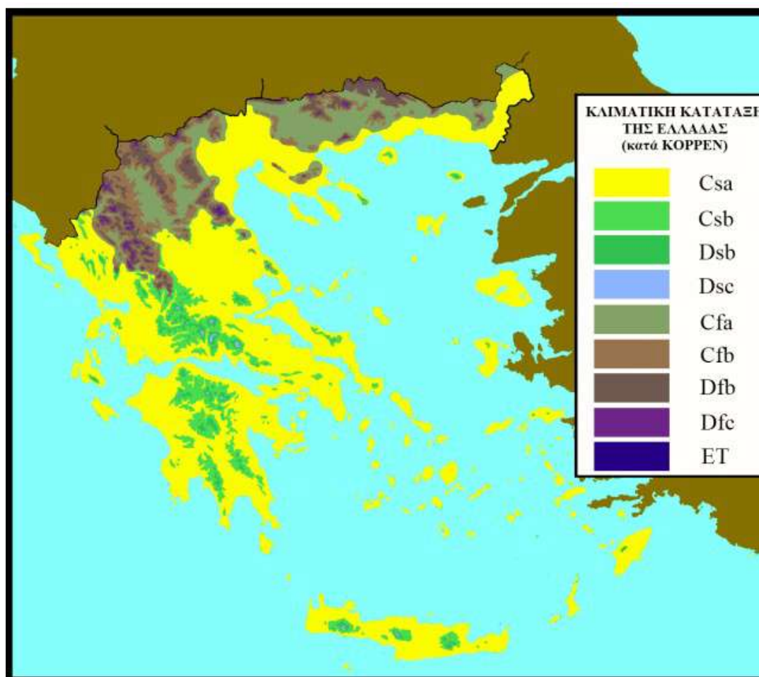
Εικόνα 2: Κλιματική κατάταξη της Ελλάδας (κατά Koppen).
