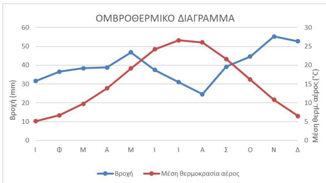
Γράφημα 4: Ομβροθερμικό διάγραμμα Μ.Σ. Κορδελιού για την περίοδο 2018 – 2023.
