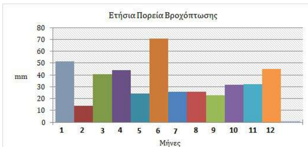
Γράφημα 1: Γραφική απεικόνιση μέσης βροχόπτωσης του Μ.Σ. Κορδελιού για την περίοδο 2018 – 2023 (Πηγή: meteo.gr).
