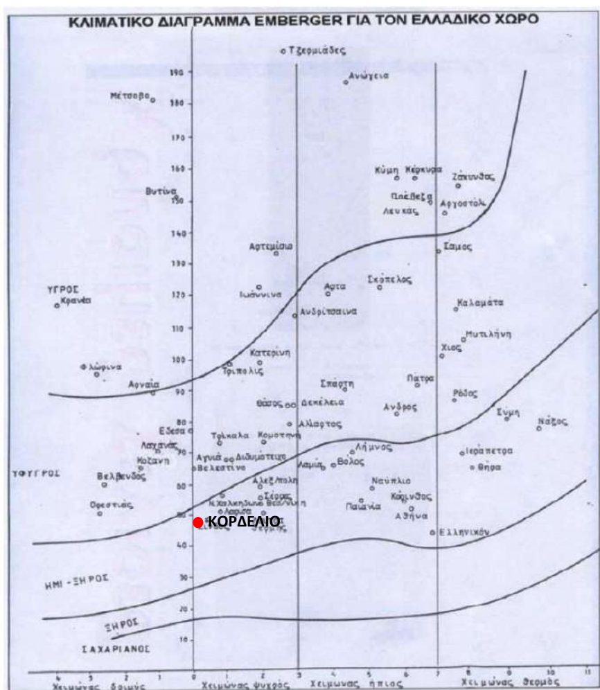
Γράφημα 5: Κλιματικό διάγραμμα Emberger για τον Ελλαδικό χώρο. Εντοπίζεται η περιοχή μελέτης.
