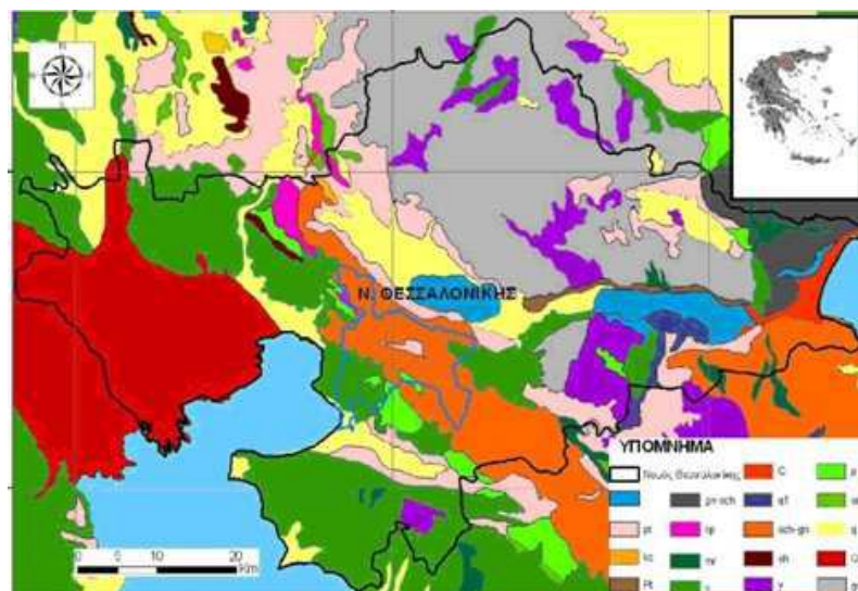
Χάρτης 3. Γεωλογικός χάρτης της περιοχής του νομού Θεσσαλονίκης
