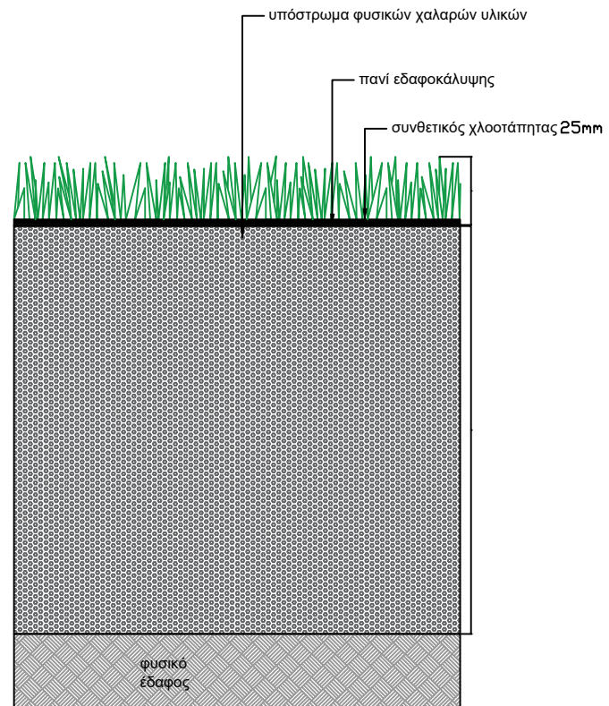
ΟΛΟΚΛΗΡΩΜΕΝΟ ΣΥΣΤΗΜΑ ΔΑΠΕΔΟΥ ΑΣΦΑΛΕΙΑΣ- ΤΟΜΗ
