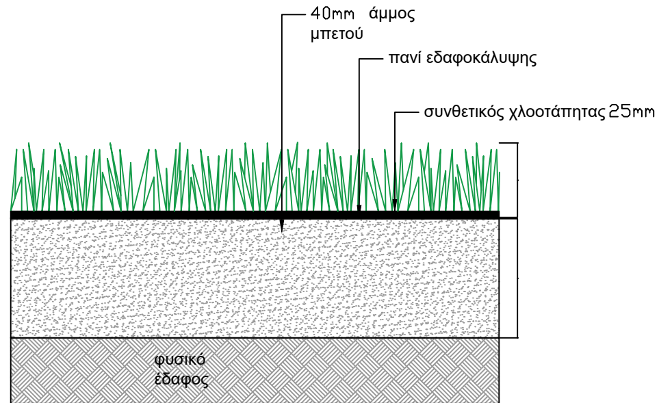
ΣΥΝΘΕΤΙΚΟΣ ΧΛΟΟΤΑΠΗΤΑΣ- ΤΟΜΗ
